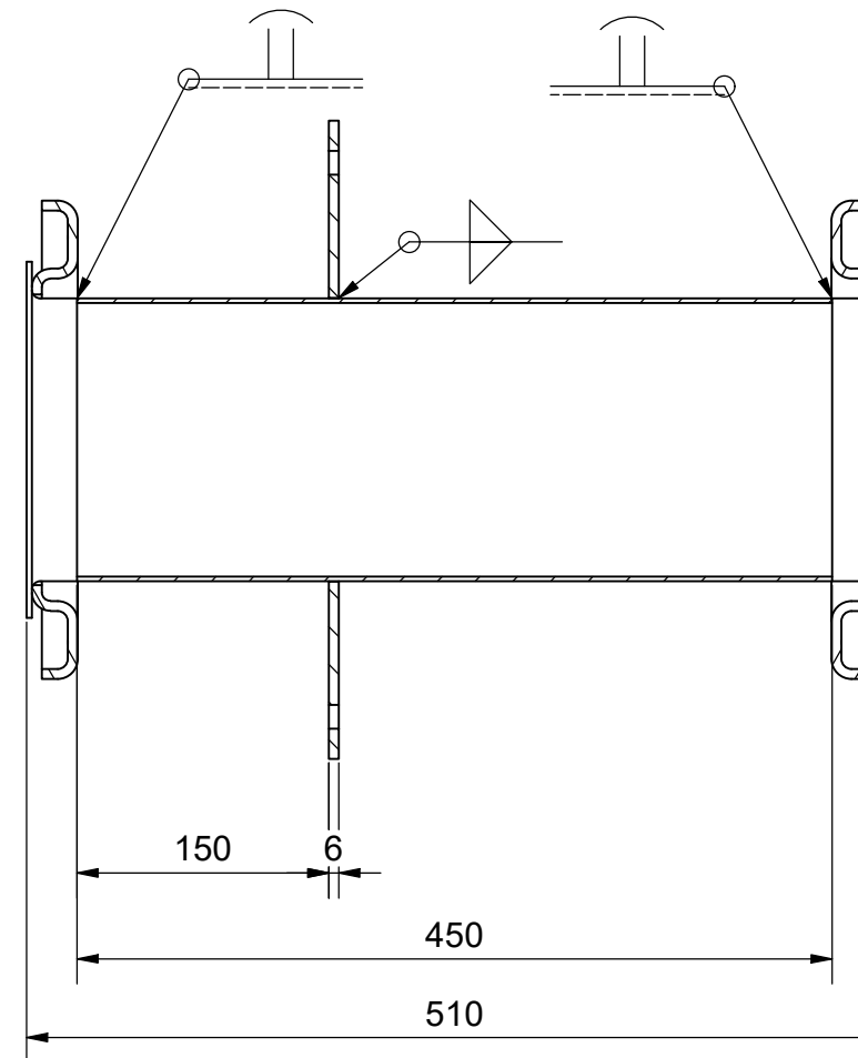
A-A ( 1 : 5 )
